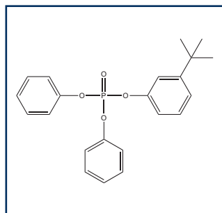
3tBPDP
